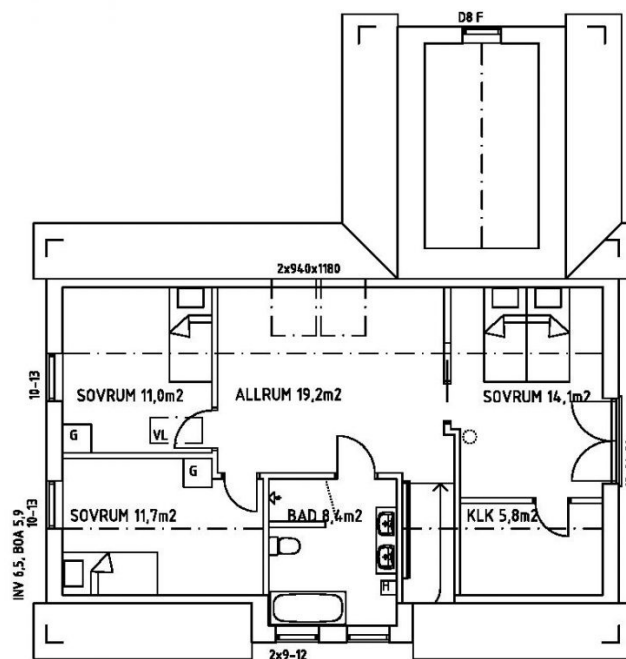
VINDSPLAN 75,9m 2 , 69,8m 2 BOAREA
