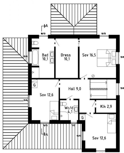
Överplan Inv. area: 88,2 m 2
