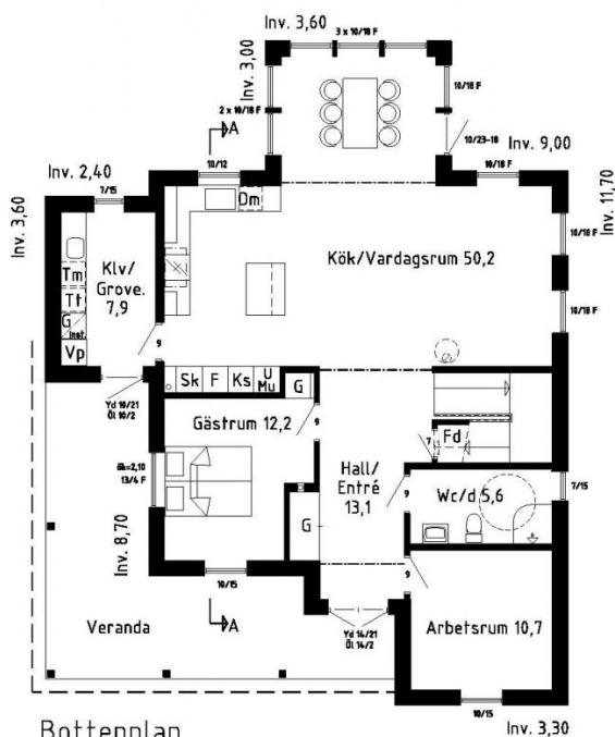
Bottenplan Inv. area: 109,5 m 2 Byggnadsarea: 156,4 m 2
