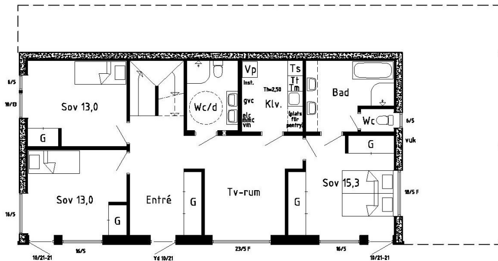
Entréplan Inv. area: 98,5 m 2
