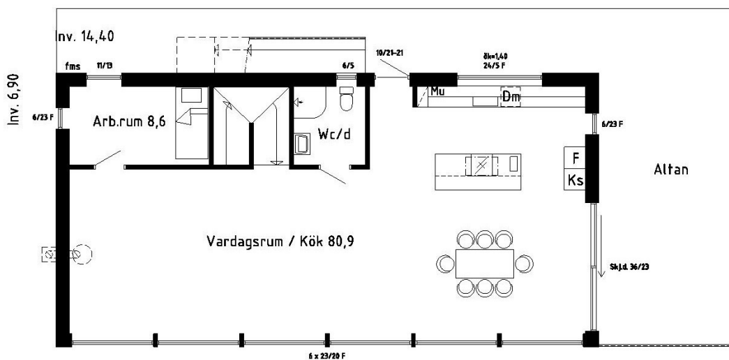
Överplan Inv. area: 99,4 m 2
