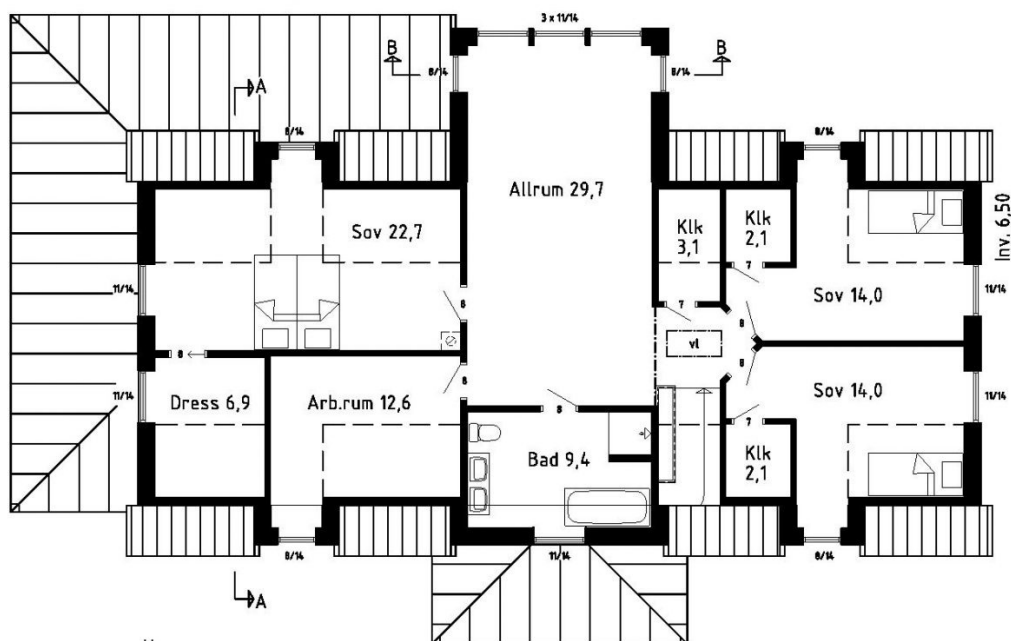
Överplan
